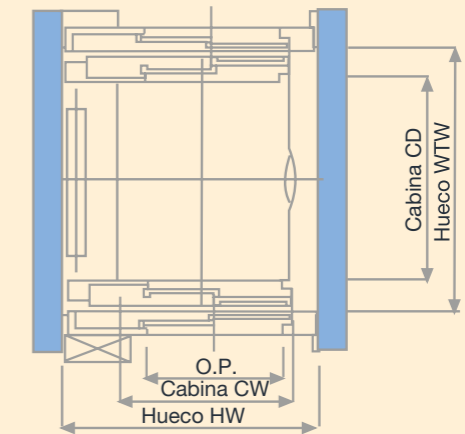
CROQUIS DE PLANTA
